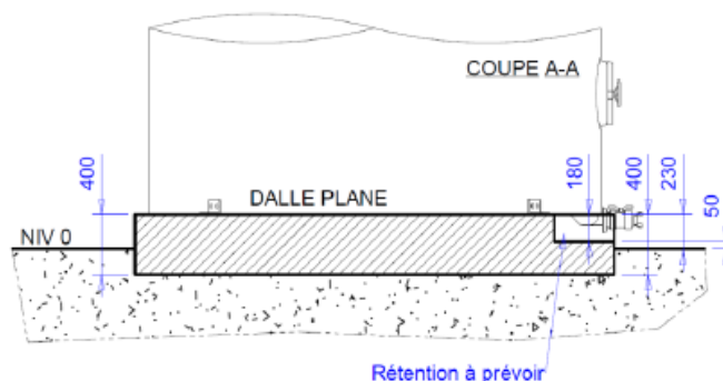
Plan de dalle pour vidange totale
