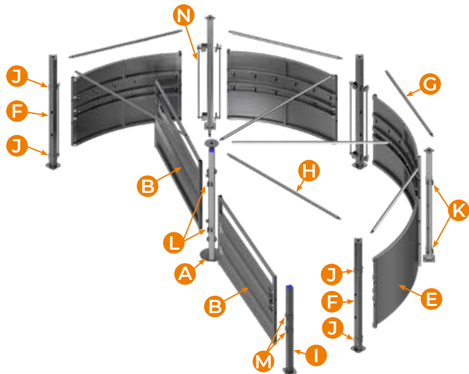
DÉTAIL 1/2 CIRCULAIRE ENTRÉE DIRECTE
