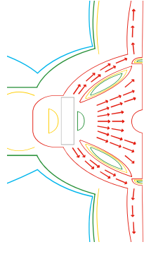
FLUX D'AIR DU CYCLONE 360
